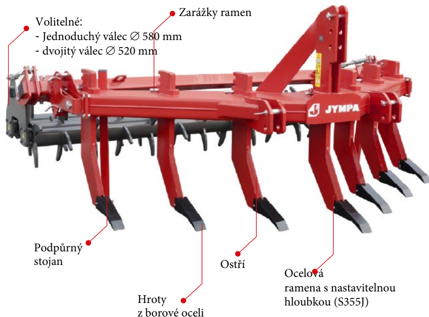
Model ANTARES-7 s dvojitým válcem Ø 520 mm
