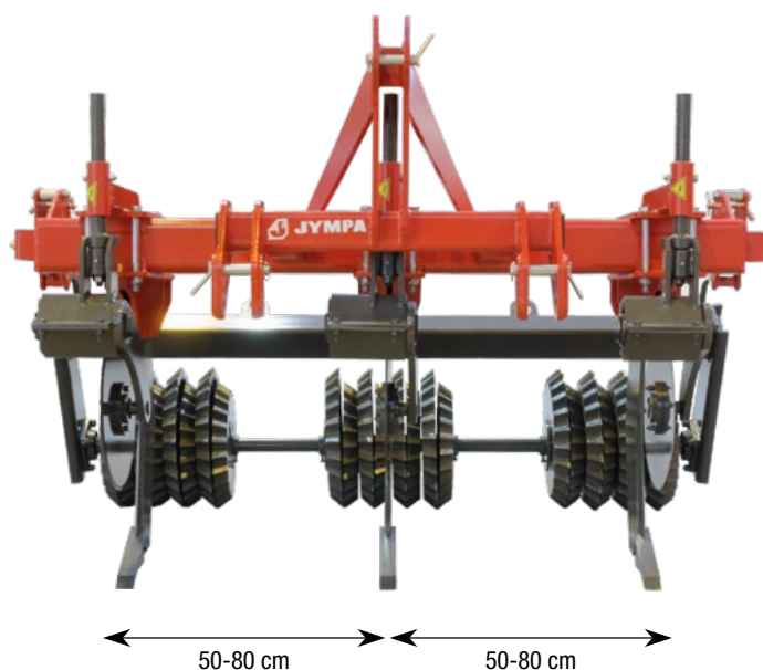
Model ALASIA-3-AR s hvězdicovým válečkem Ø 500 mm a s mechanicky nastavitelnou vzdáleností mezi rameny
